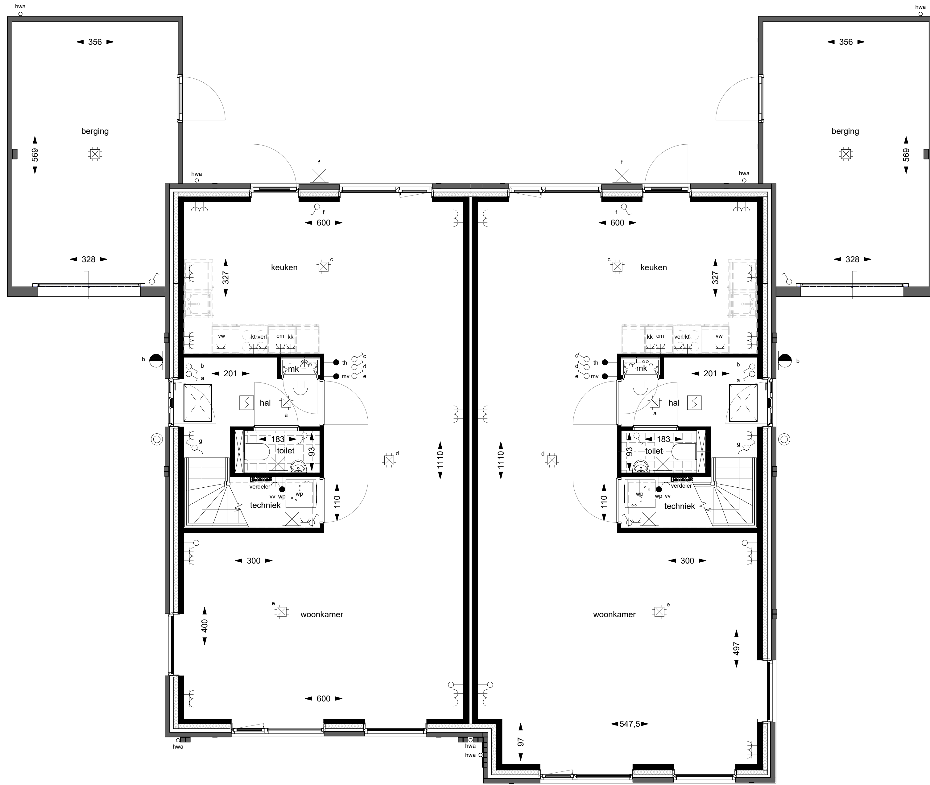
Begane grond bouwnummer 1 en 3
