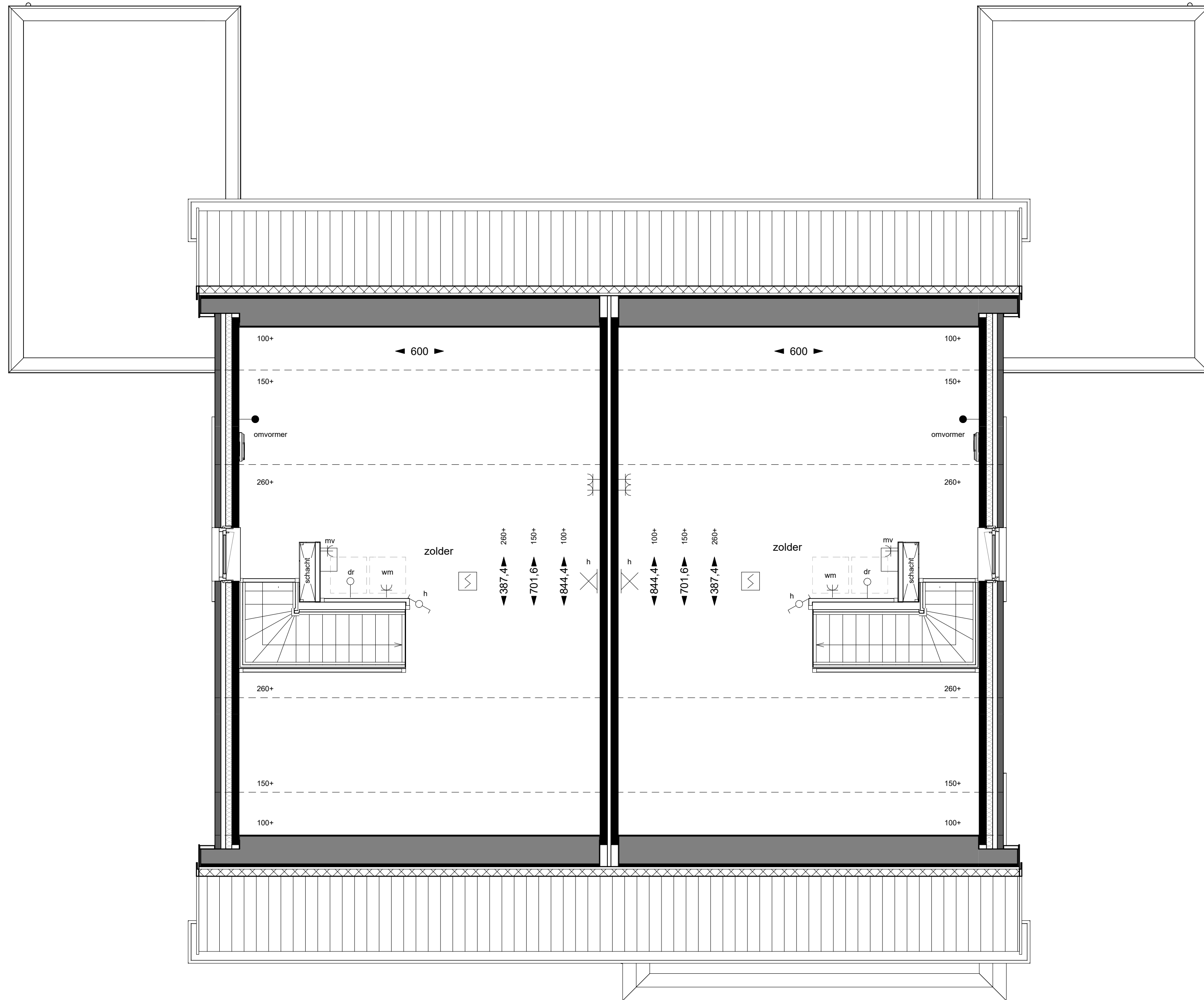
2e Verdieping bouwnummer 1 en 3
