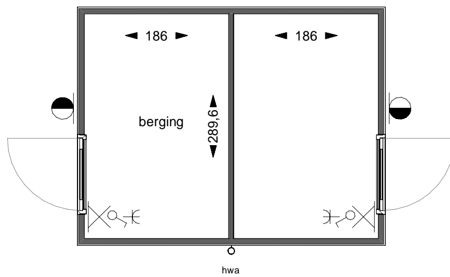
Plattegrond 1:50
